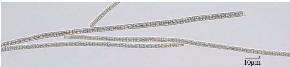
图1 HAB631阿氏浮丝藻
